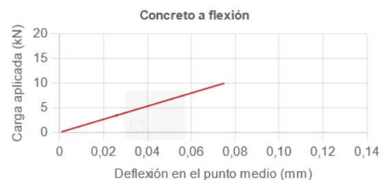
Figura 1: Carga aplicada a la viga en kN vs deflexión en el punto medio.
